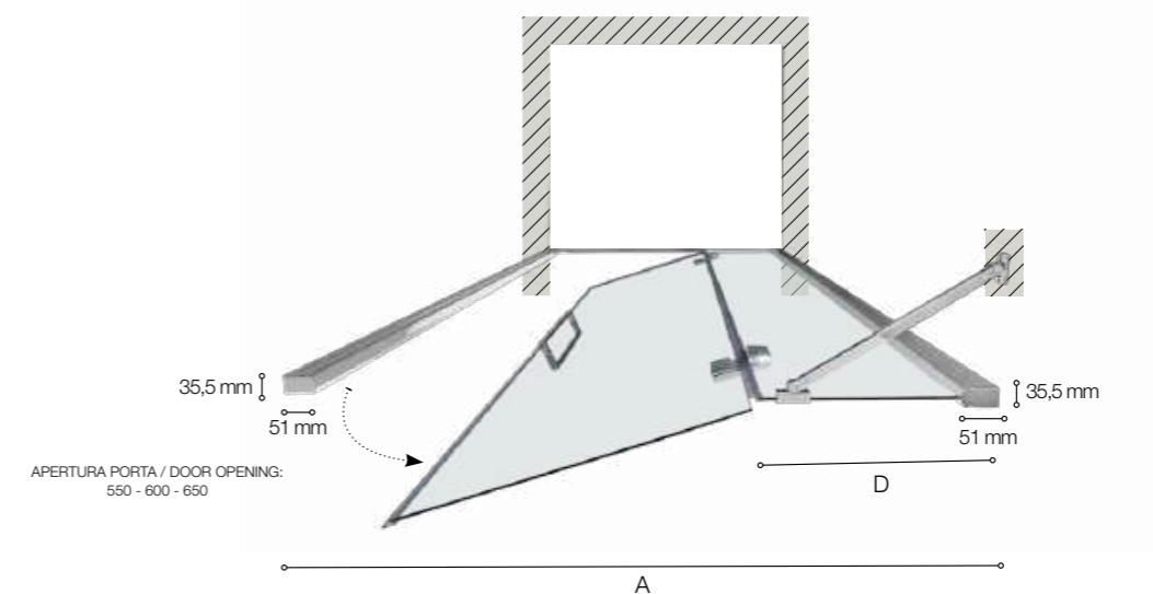
DIMENSIONI PORTA (A) (NICCHIA) CON PROFILO DI CHIUSURA NTPC01 DOOR SIZE (A) (NICHE) WITH CLOSING PROFILE NTPC01
