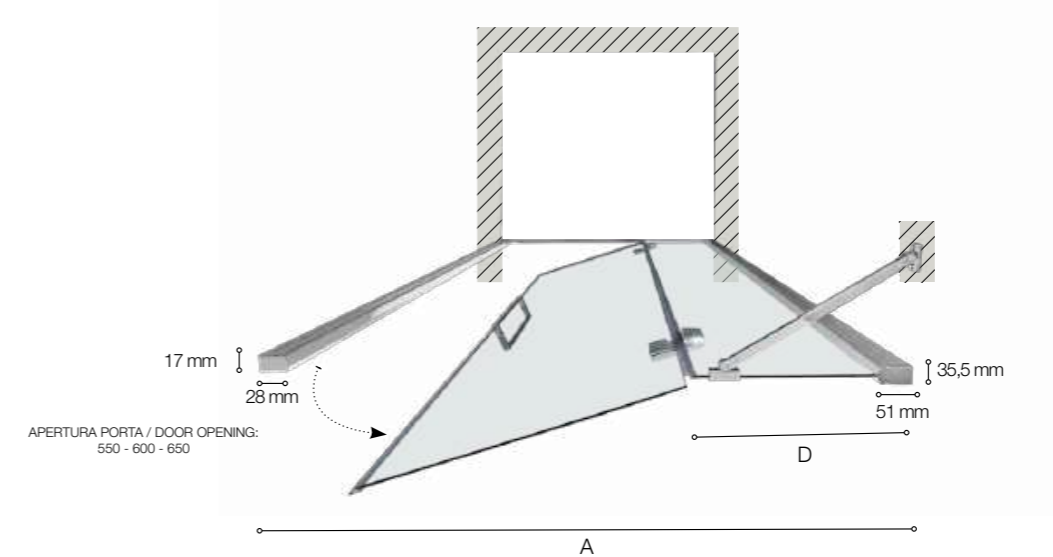
DIMENSIONI PORTA (A) (NICCHIA) CON PROFILO DI CHIUSURA NTPC03 DOOR SIZE (A) (NICHE) WITH CLOSING PROFILE NTPC03
