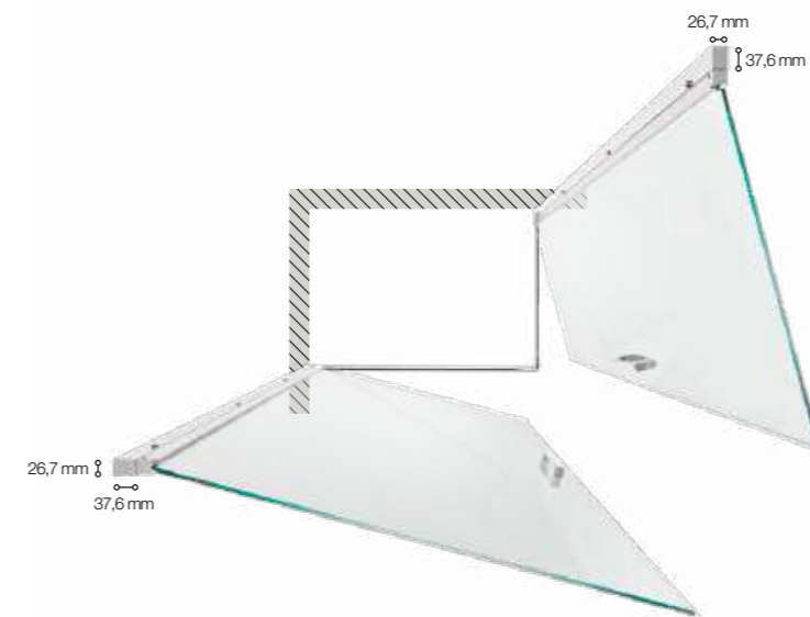
DIMENSIONI DOPPIA PORTA (A) DOUBLE DOOR SIZES (A)
