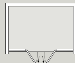
Doppia porta battente Versione: Nicchia
