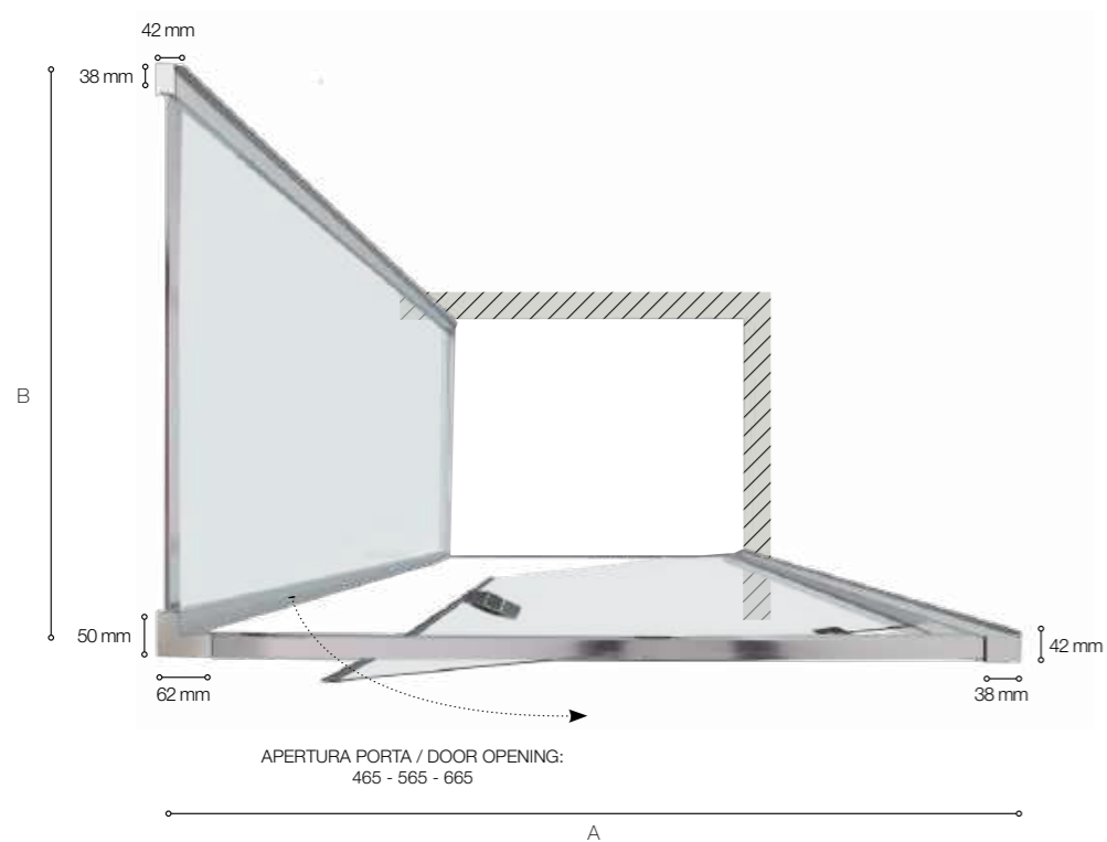
Versione Angolare DX da 90 cm Right Corner Version 90 cm
