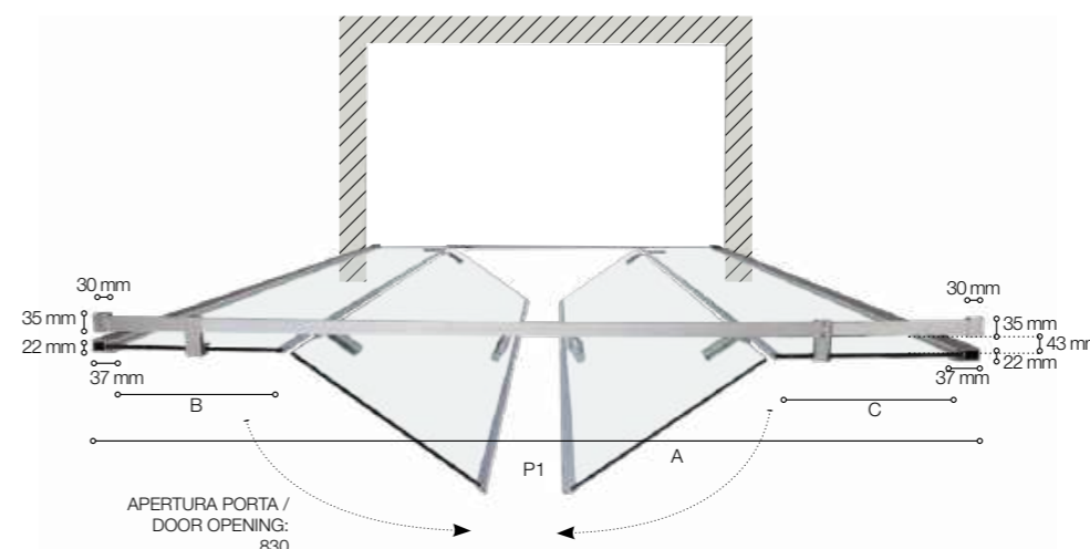
Versione nicchia Niche version
