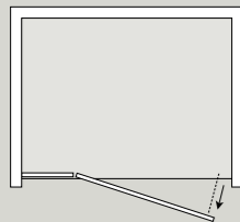
Porta battente Versione: Nicchia Hinge door Version: Niche
