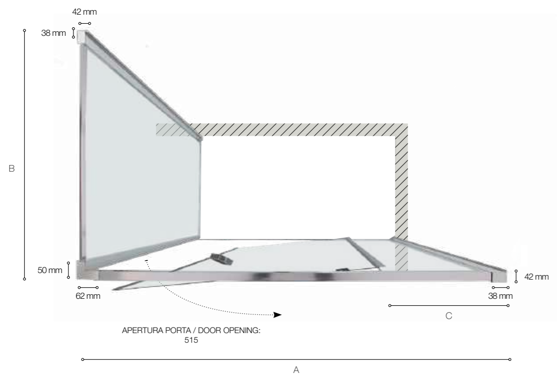
Versione Angolare DX da 120 cm Right Corner Version 120 cm
