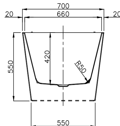
SEZIONE G-G
