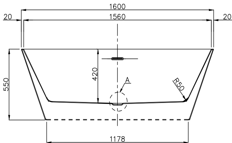
SEZIONE F-F
