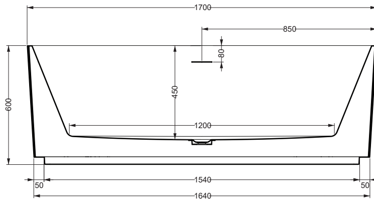
SEZIONE LONGITUDINALE
