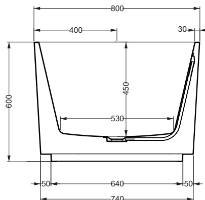
SEZIONE TRASVERSALE
